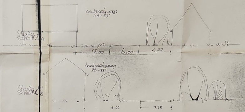
Straßenquerschnitte M 1 = 1/200
